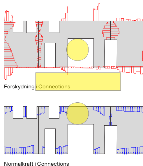
Figur 5.3.1 Lastdata udtaget fra en elastisk FEM-model
